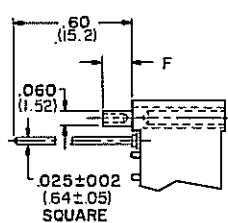
Wrapping
